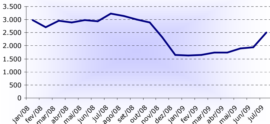
Produção de Aço Bruto - Brasil - Julho de 2008 a Julho de 2009 - unidade: 10 3 T.
